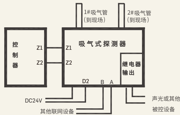
接线示意图
