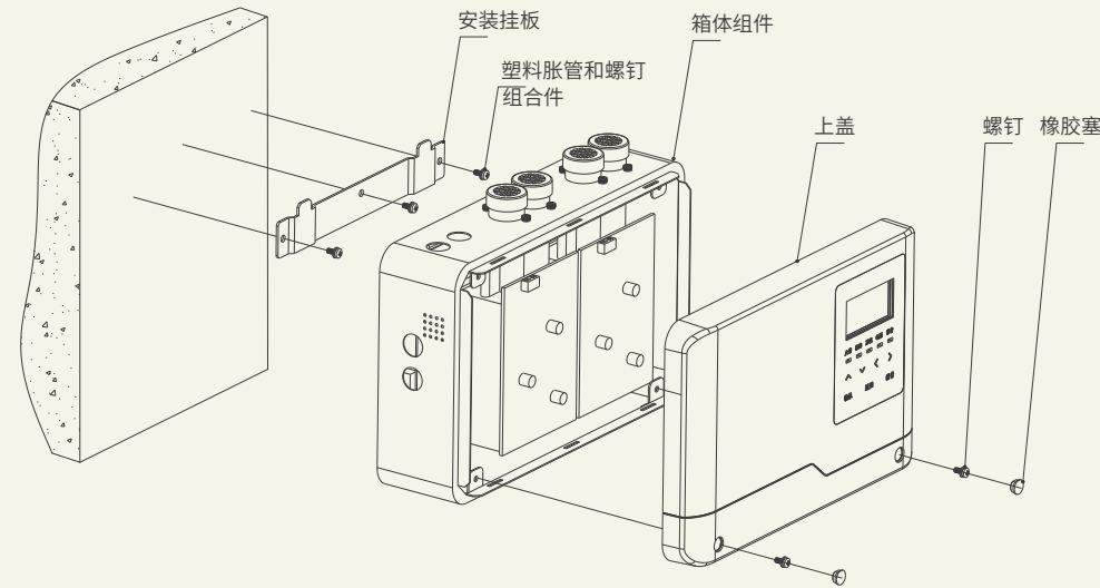
JTY-GXF-GST2D安装示意图
